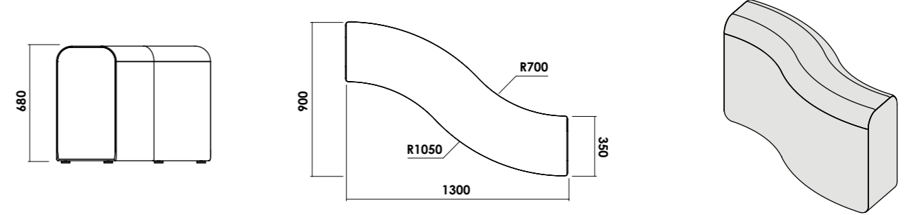
XOS-L-2600 XOXO LOOSE - CHICANE LHS PERCH
