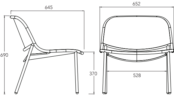
Lounger 652w x 645d x 690h
